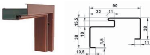
OŚCIEŻNICA ASYMETRYCZNA Z USZCZELKĄ FA (do drzwi TT, GTT)
