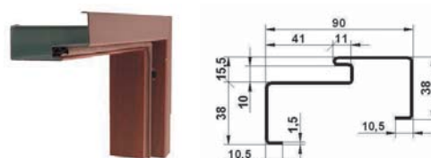
OŚCIEŻNICA ASYMETRYCZNA Z USZCZELKĄ FA (do drzwi TT PLUS, TT MAX, GTT PLUS, GTT MAX)
