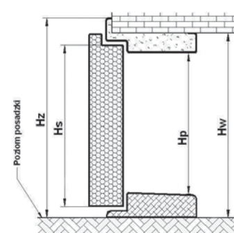
Ościeżnica drzwi, próg
