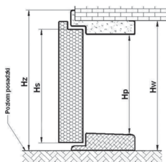
Ościeznica drzwi, próg
