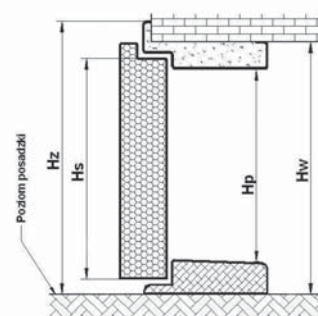
Ościeżnica drzwi, próg
