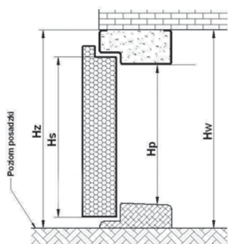
Ościeznica drzwi, próg
