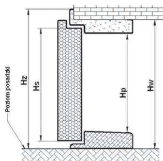
Ościeznica drzwi, próg
